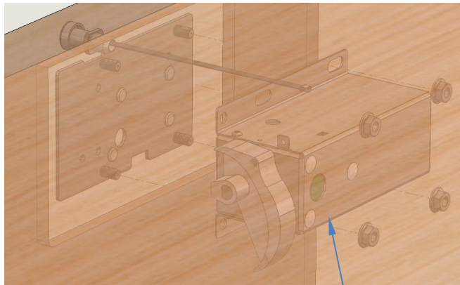
Zuziehgehäuse
