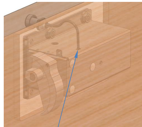
Sensorkabel
