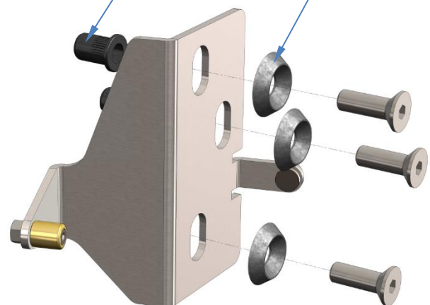
Senkscheibe
