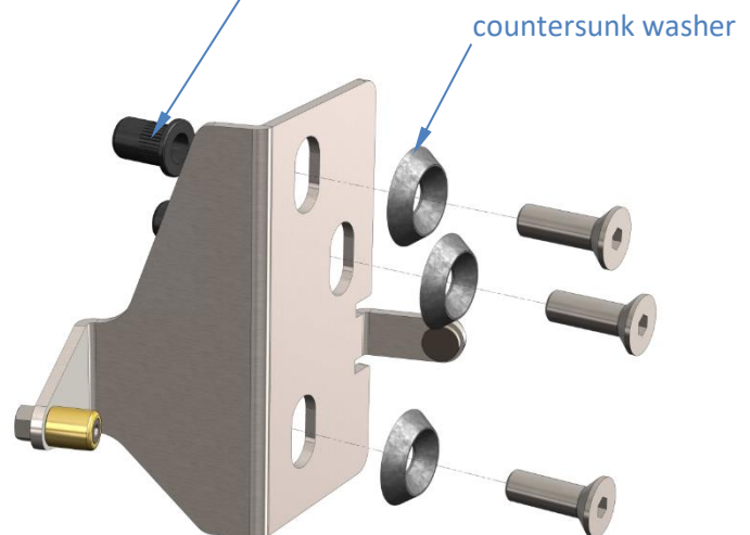
rivet nuts
