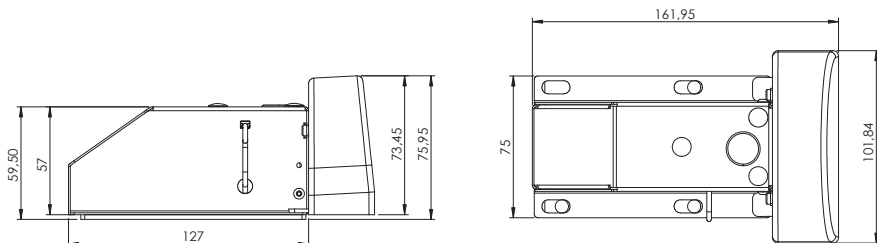
Abmaße Baugruppe Motor SC1.1 Malibu
